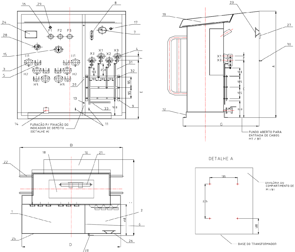
Figura 5 - Transformador pedestal em anel
