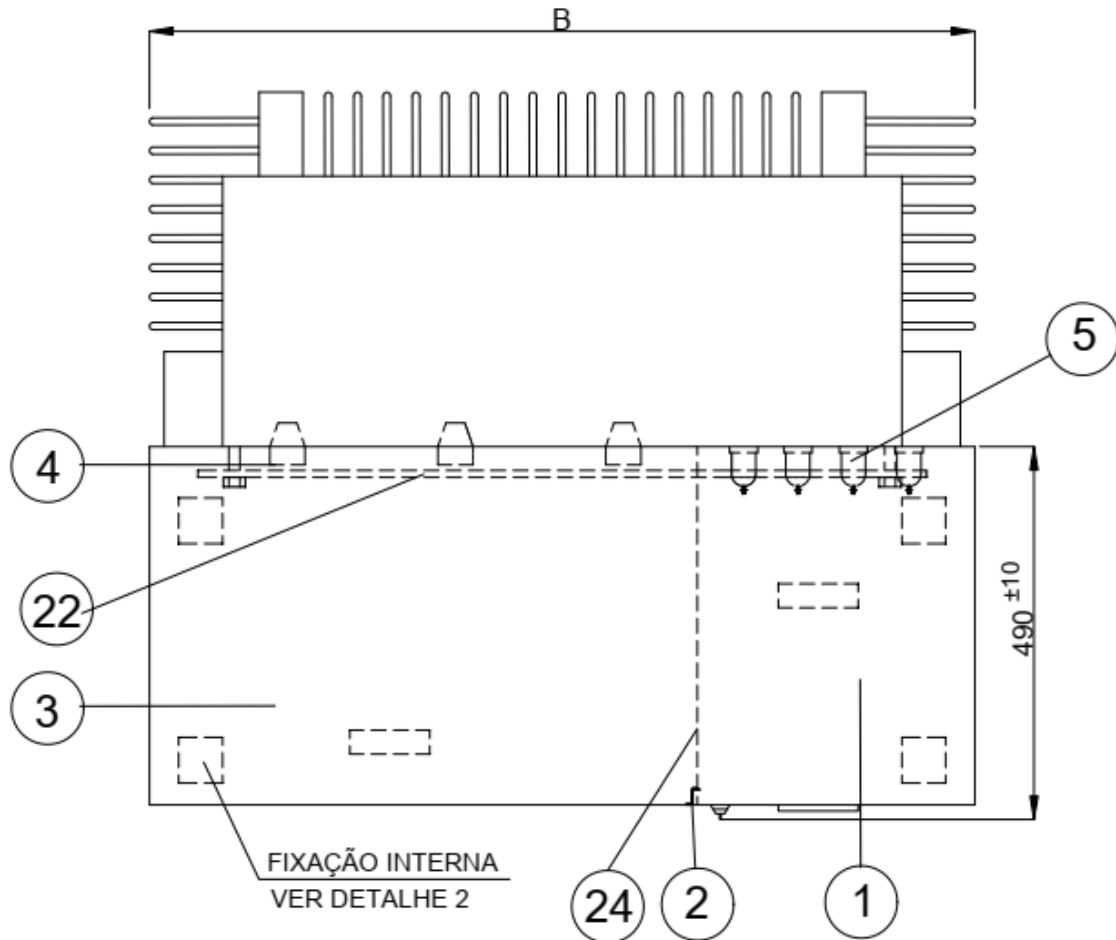
Figura 3 - Transformador pedestal radial – vista superior
