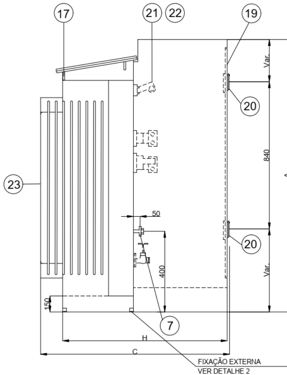
Figura 2 - Transformador pedestal radial – vista lateral
