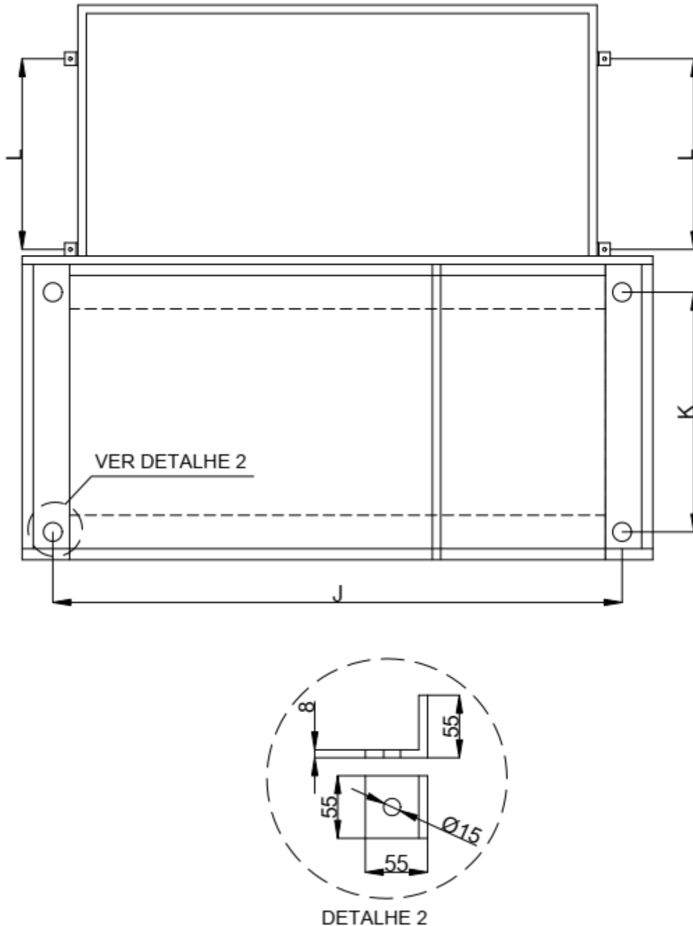
Figura 4 - Transformador pedestal radial - vista inferior
