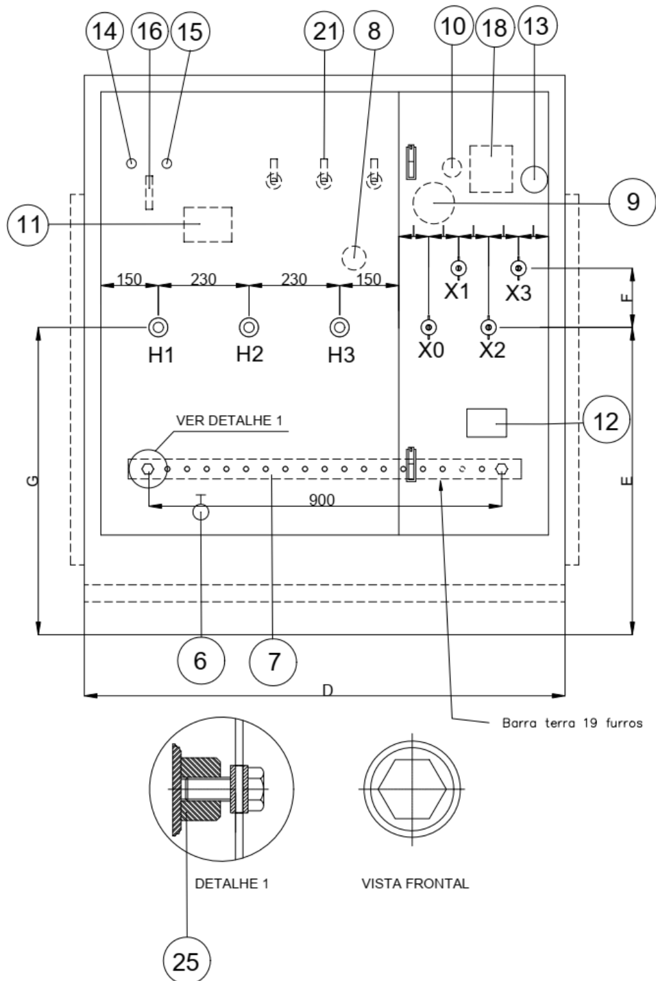
Figura 1 - Transformador pedestal radial - vista frontal
